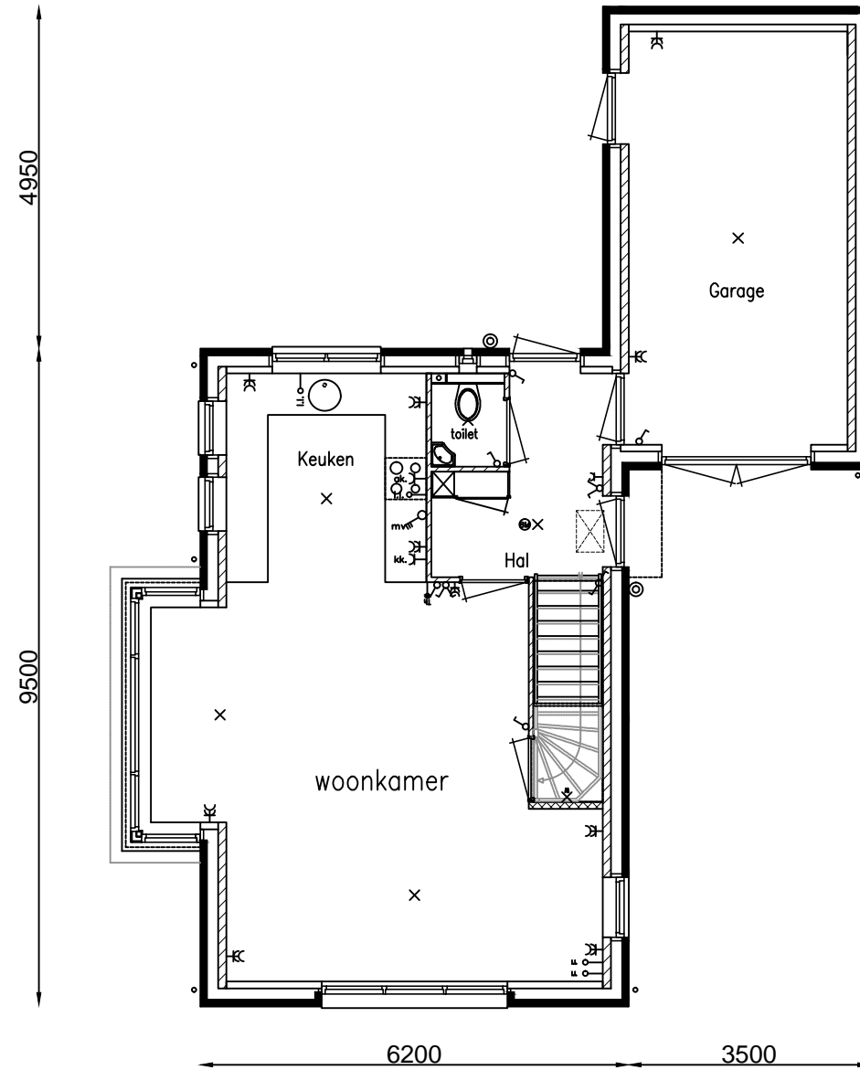
begane grond (schaal 1:100)
