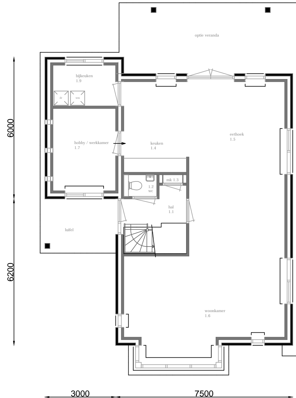
begane grond (schaal 1:100)
