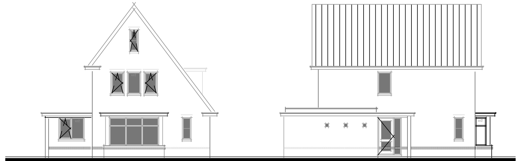
voorgevel
